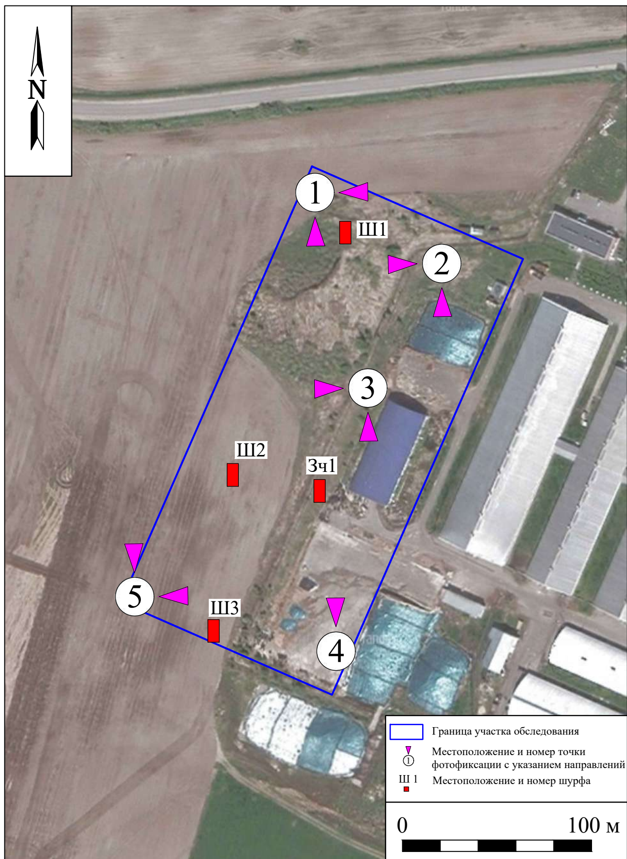
Рис. 7 . Археологические разведки в Кстовском р-не Нижегородской области. 2026 г. Ситуационный план участка обследования с указанием местоположения шурфов, точек фотофиксации и их направлений на космоснимке 2025 г.
